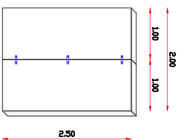
Fixation avec un fer plat acier Hauteur = 2.50
