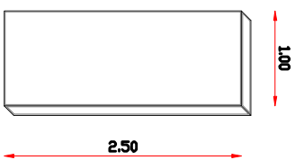
Cloison type C (1.00 X 2.50) Epaisseur = 6cm
