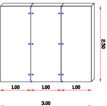
Fixation avec un fer plat acier Hauteur = 3.00
